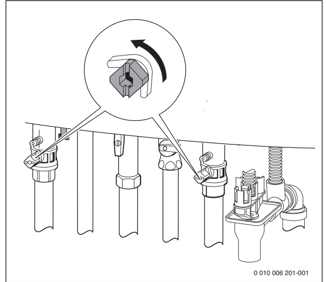
Мал. 3 Відкриття кранів для техобслуговування
